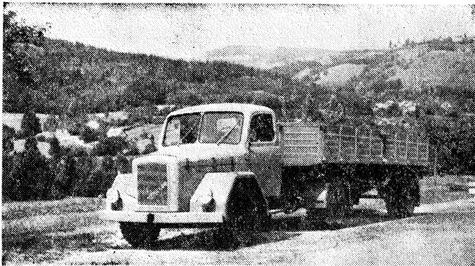
Kamion-vlačilec »TAM 4500 VL«
