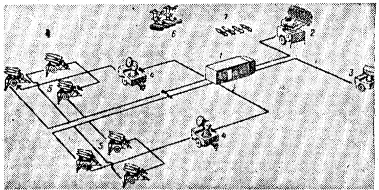
BOJNA RAZPOREDITEV RAKETNE ENOTE: 1 — komandno mesto; 2 — opazovalni radar za visoke cilje; 3 — opazovalni radar za nizke cilje; 4 — radar za »osvetljevanje« cilja; 5 — izstrelišča raket; 6 — parkirišče za transportna vozila; 7 — skladišče raketnih izstrelkov
