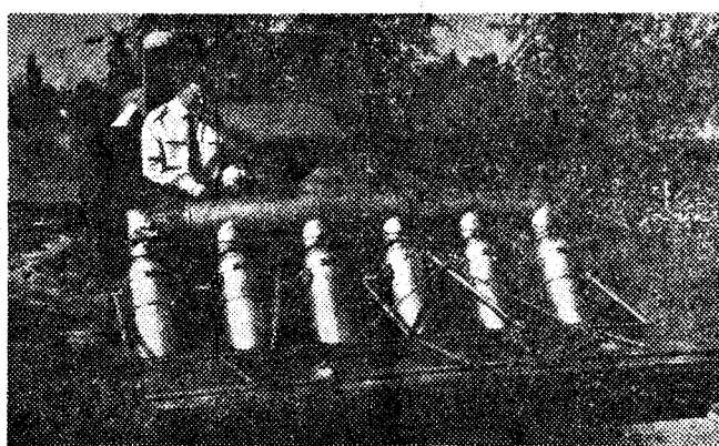
NAPRAVA ZA TOPITEV SNEGA na vzletnih stezah je izum kapetana Josipa Vodopivca, razstavljen pa je bila tudi na mednarodni razstavi izumov v Bruslju. Ob tej priložnosti je kapetan Vodopivec zanj prejel zlato medaljo in diplomu. Na sliki vidimo izumitelja zraven svojega topilca snega.
