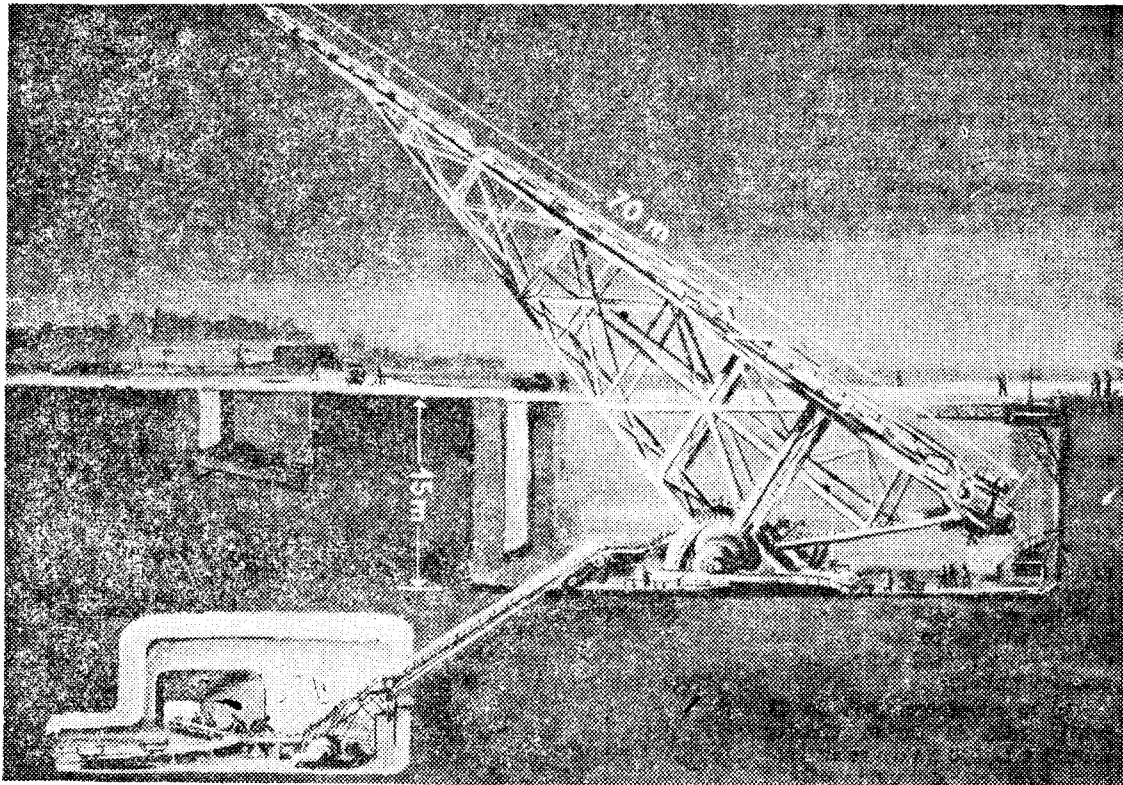
Električni top kal. 150 mm in z dosegom 250 kilometrov
