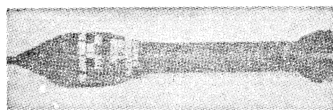
BELGIJSKI ROČNI METALEC »BLENDICIDE«, ki ga vidimo na sliki, je zelo uspešen proti vsem oklopnim vozilom. Poročajo, da njegova 2,75 kg težka mina, ki leti do 220 m daleč, lahko prebije 40 cm debel jeklen oklep.
