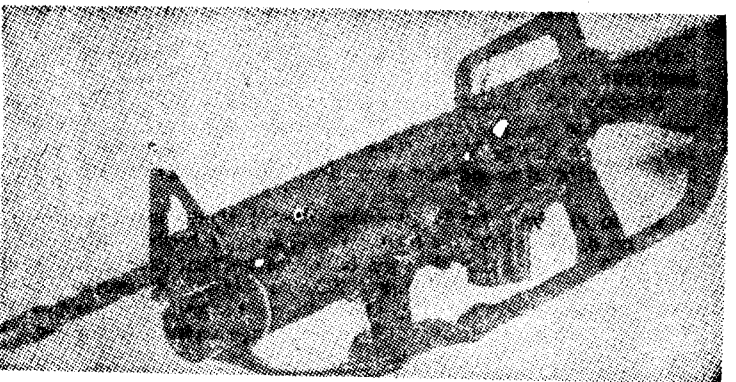
Avtomatska puška M 16 s cevjo XM 148 (kal. 40 mm)
