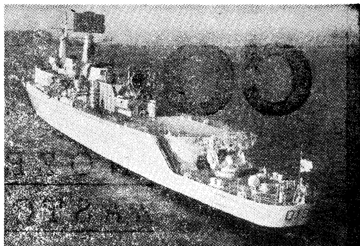
Na sliki vidimo najnovejšo britansko raketno fregato »Glamorgan«, kakršnih imajo Angleži že šest. V sredini ladje je parabolični žaromet radarja za usmerjanje raket »Seaslug« na cilj, antena na jamboru pa pripada artiljerijskemu radarju
