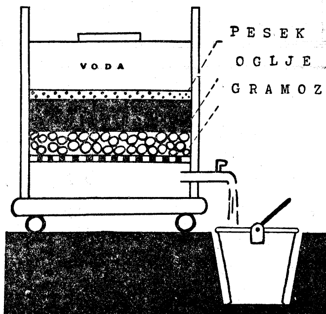
Presek cedila za čiščenje vode
