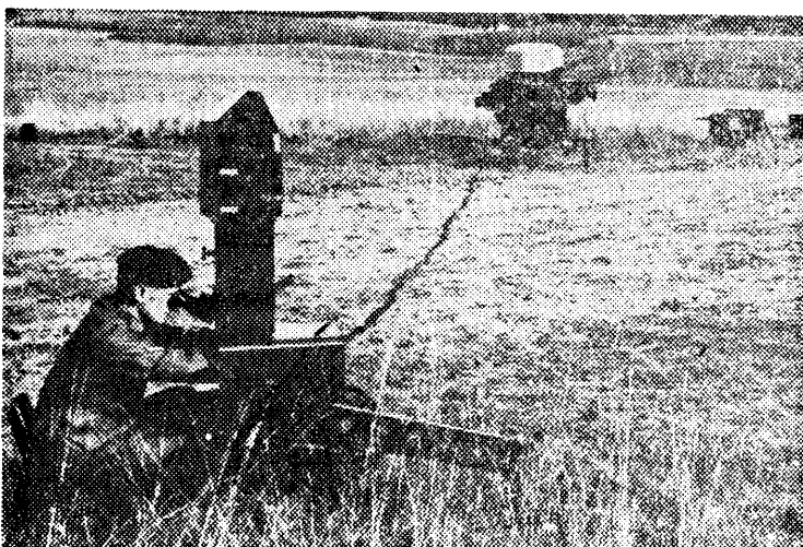
NA SLIKI VIDIMO VSE TRI ELEMENTE SISTEMA »RAPIER«: NA LEVI STRANI JE NAPRAVA ZA USMERJANJE, V SREDINI PODSTAVEK Z RAKETAMI IN RADARJEM, DESNO OD NJEGA PA GENERATOR
