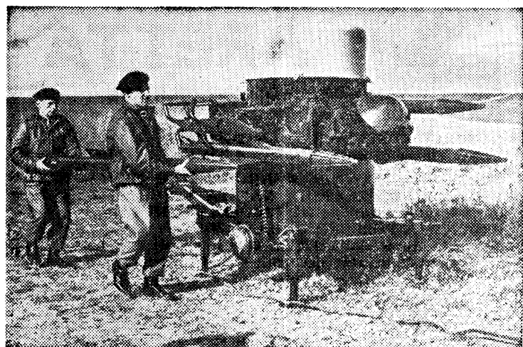
VRTLJIVI PODSTAVEK S STIRIMI RAKETAMI, KI SO DOLGE PO 224 CENTIMETROV, LETE PA S HITROSTJO DO 2400 KILOMETROV NA URO
