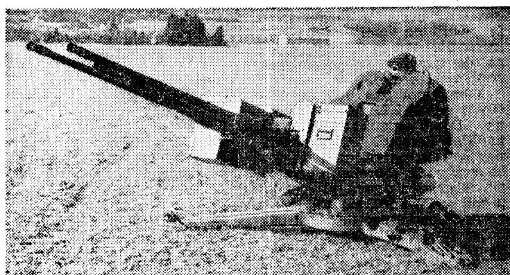
AMERIŠKI TRICEVNI TOP 20 MM HSS 635 JE NAMENJEN ZA OBSTRELJEVANJE CILJEV V ZRAKU IN NA TLEH
