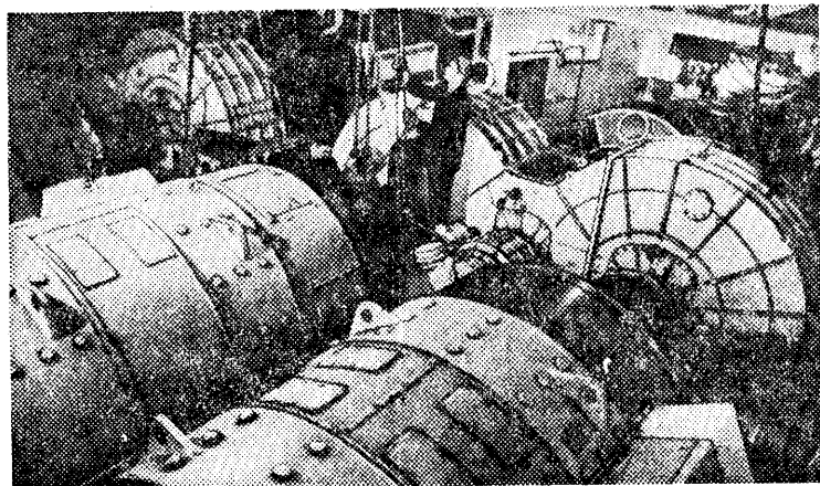
Strojnica atomske ladje »Lenin«
