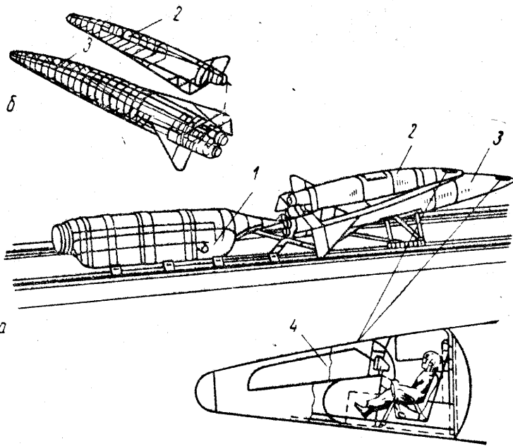
RAKETA-NOSILKA ZA VEČKRATNO UPORABO: a — OB VZLETU; b — RAZDVOJITEV; 1 — PRIKOLICA NA TRAČNICAH Z GORIVOM; 2 — DRUGA STOPNJA; 3 — PRVA STOPNJA; 4 — KABINA ZA POSADKO
