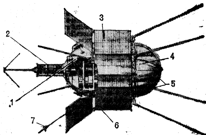
SOVJETSKI SATELIT »KOSMOS 97«: 1 — ZNANSTVENI APARATI; 2 — JEDRSKI GENERATOR; 3 — SONČNE CELICE; 4 — BATERIJE; 5 — TERMOSTAT; 6 — PROSTOR ZA OPREMO; 7 — DETEKTOR ZA KONTROLNO VIŠINE
