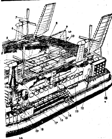
Britanski aerogliser SR.N.4: 1 — kabina za krmarja; 2 — stopnice do krmarjeve kabine; 3 — odprtine za zrak; 4 — ventilator za potniške kabine; 5 — cevi za toplotne kabele; 6 — loputnica turbinskega oddelka; 7 — vijaki; 8 — pomožni motorji za električno energijo; 9 — zadnja vrata; 10 — prostor za tovor; 11 — odprtine za dovod zraka k turbini; 12 — turbine; 13 — rešilni čoln; 14 — gonilna os; 15 — rezervoarja; 16 — stopnišče za posadko; 17 — ventilatorji za potniške kabine; 18 — dva metra debela zunanja stena; 19 — rampa za iztovarjanje.
