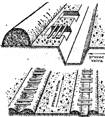
Zasilno ognjišče za menažke
