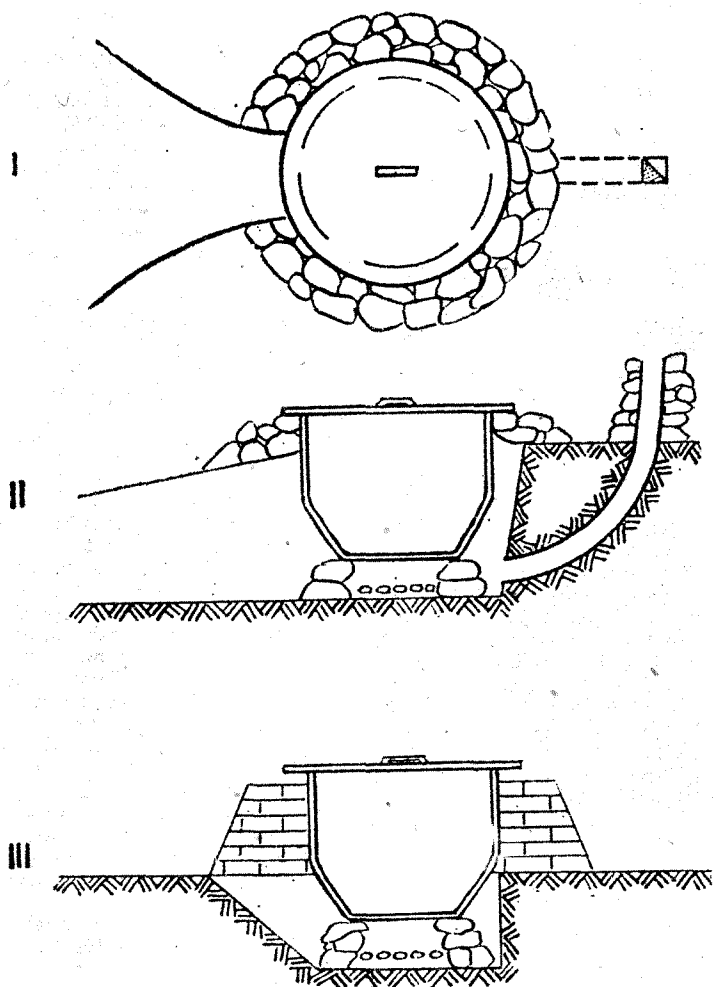
Napol vkopano ognjišče za kotel: I — pogled od zgoraj, II — presek po dolžini, III — pogled s prednje strani.
