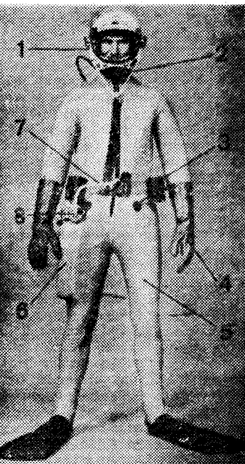
POTAPLJAC V TERMOKOMBINEZONU Z ELEKTRICNIM GRETJEM 1 — potapljaška čelada, 2 — krožni podstavek za čelado, 3 — akumulator, 4 — rokavice, ki so tudi na električno gretje, 5 — vrhne zaščitno oblačilo iz gobastega neoprena, 6 — steklenica s stisnjenim zrakom (ali neonom), 7 — cev za vzdrževanje enakega pritiska v obleki, 8 — regulator za jakost gretja.
