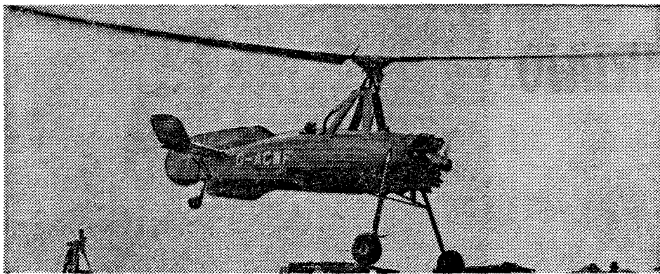
Avtožir španskega inženirja Juana de La Cierva iz leta 1923. Avtožir je letalo, ki ima namesto kril rotor, ki ga ne poganja motor, ampak zračna struja. Zato avtožir potrebuje za pristajanje in poletanje prav tako kot letalo večji prostor
