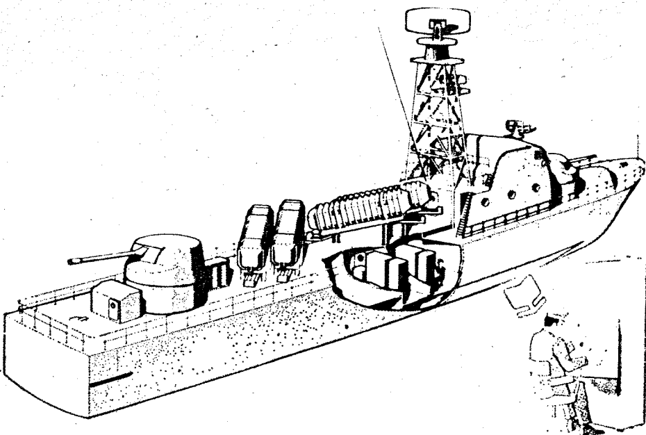
Samo en sam operater na motorni topničarki tipa kimotoi zadostuje, da lansira raketo exocet in jo vodi proti cilju.
