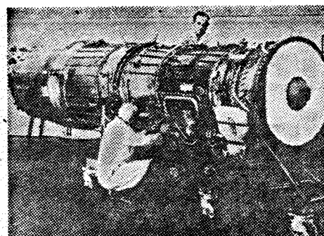
Reaktor Floo se odlikuje ne le po izredno ugodnem razmerju med močjo in težo (9:1), ampak tudi po konstrukciji, ki olajšuje vzdrževanje in zamenjavo posameznih delov.
