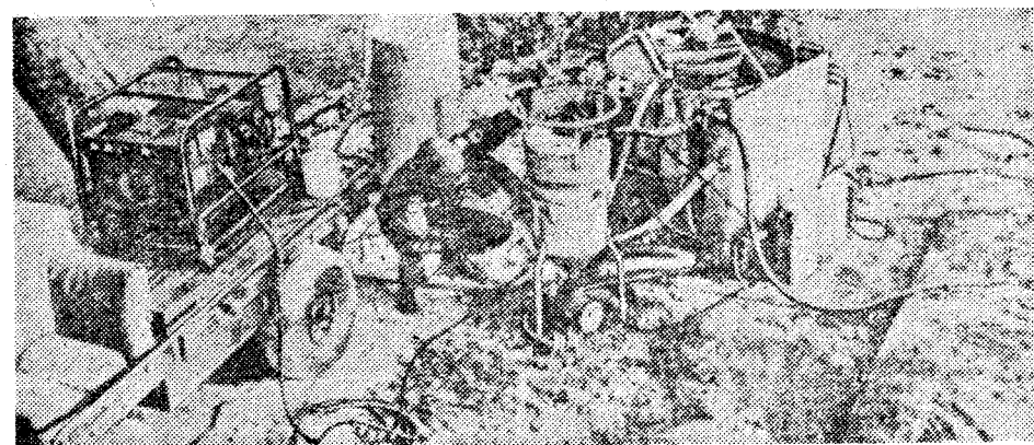
Lahka terenska naprava za čiščenje vode, kakršno uporablja nemška armada.
