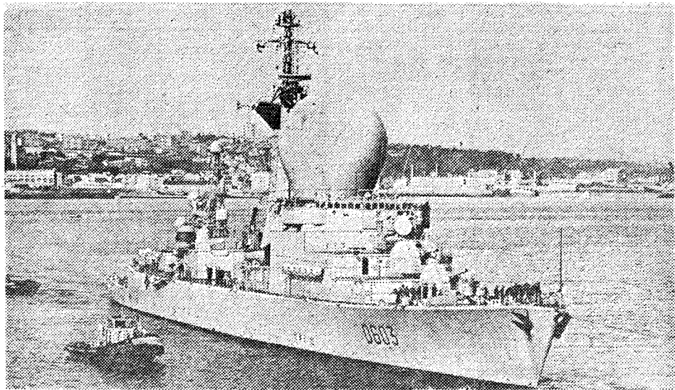
Raketna fregata 603 DUQUESNE tipa FLM 60, ki je bila zgrajena pred petimi leti, v vojno mornarico pa so jo vključili leta 1970.
