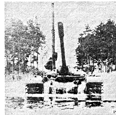
T-54 B med vajo pri premagovanju globokih vodnih ovir; levo od topovske cevi je lepo videti pokonci postavljeno cev šnorkla, po katerem dobiva tank — ko je na dnu jezera ali reke — zrak.
