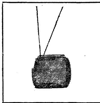
Črno-beli prenosni televizor Iskra MINIRAMA: v sodobni polvodniški tehniki s tran- zistorji in integriranimi vezji na ti- skani enoti, VHF in UHF kanalnik, priključitev na 220 V, ali akumula- tor 12 V, teža 7,5 kg, ekran 31 cm
