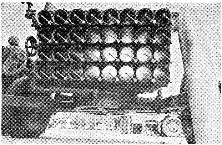
Dvaintrideset (praznih) cevi večcevnega raketometu M. 63 kal. 128 mm. Zelo dobro je videti udarne igle.
