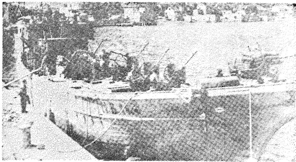
NB-11 »Crvena zvezda«, naša največja in najmočnejše oborožena ladja v NOV na morju
