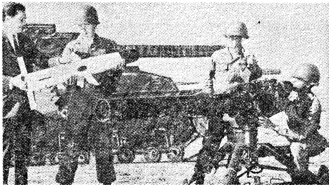
Z leve proti desni: Leta 1965 je Zahodna Nemčija začela s serijsko proizvodnjo svoje po žici vodene protitankovske rakete COBRA. Težka je dobrih 10 kg, z njo ravna en sam vojak, prebije pa 475 mm debel tankovski oklep. — TOW je težja žično vodena protitankovska raketa. Izstrelijo jo iz cevi na trinožniku, na prvi pogled podobne netržajnemu topu, lahko pa jih tudi montirajo na helikopterje. — Srednji protitankovski raketni sistem DRAGON, izdelek ameriške firme McDonnell Douglas.
