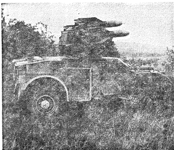
Z leve proti desni: Francoska protitankovska raketa SS-11 spada v prvo generacijo tovrstnih vodenih izstrelkov. Na sliki vidimo oklepni avtomobil NA-2, ki ima na strehi pripravljene za izstrelitev 4 rakete SS-11. — Francosko-zahodnonemška protitankovska raketa MILAN s polavtomatskim usmerjevalnim sistemom, ki ima učinkovit dolet do 2000 metrov. — Razvoj protitankovskih raket ni skokovit. Na fotografiji je helikopter, oborožen s 6 francosko-zahodnonemškimi protiletalskimi raketami HOT, ki imajo polavtomatsko usmerjanje in dolet 4000 metrov.
