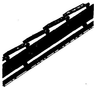
strešna opaba vodotesna strešna lepenka leseni škarniki (špirovci)
