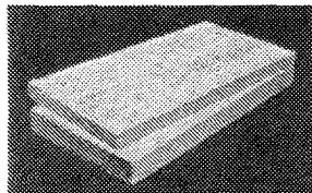
Plošče iz kamene volne Tervol vezane s fenoplastom, za ognjevarno izolacijo raznih konstrukcij, zračnih kanalov.
