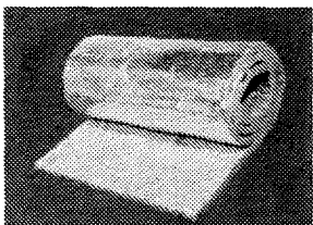
Elastični filc iz kamene volne Tervol, vezan s fenoplastom, enostransko obložen s aluminijasto folijo (parna zavora), za toplotno in zvočno izolacijo
