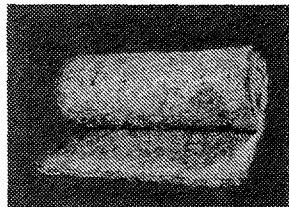
Elastični filc iz kamene volne Tervol vezan s fenoplastom, za toplotno in zvočno izolacijo podov, stropov, sten in strešnih delov z oblogami. V industriji za izolacijo podov, kotlov, cevi itd.
