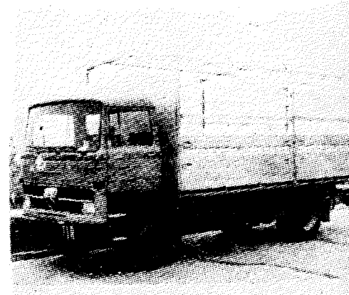
Palletna TIR nadgradnja na vozilu MB 1113(1213)
