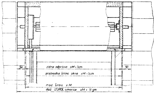
Načrt roletne omarice »Izorol«
