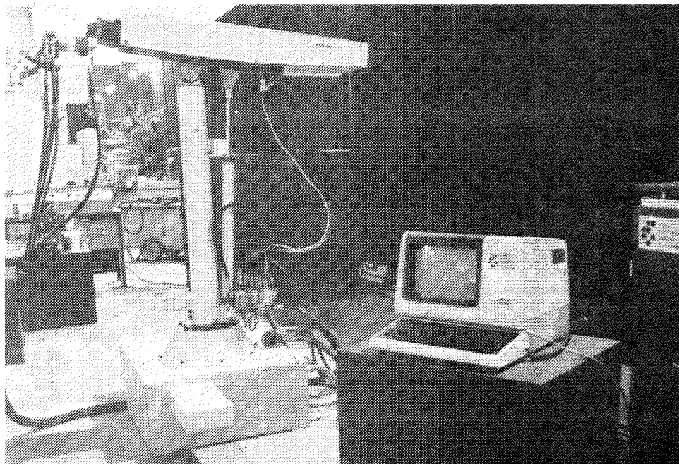
Robot za nanašanje emajla, lakov in barv z brizganjem
