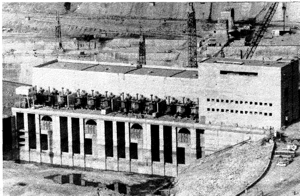
Največji objekt, pri katerem je kdajkoli sodelovala Hidromontaža, je bila izgradnja hidroenergetskega in namakalnega sistema Tarbela Dam v Pakistanu. Na fotografiji je strojnica hidroelektrarne.
