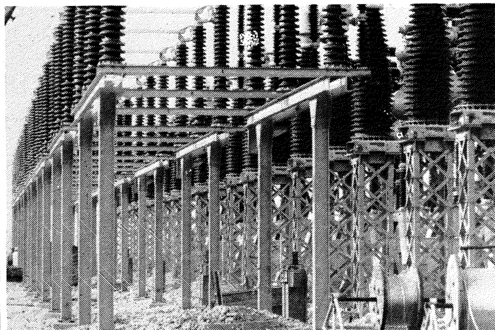
Pogled na stikala 220 kV stikališč
