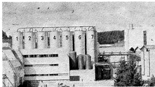
Silos za shranjevanje surovin za proizvodnjo antibiotikov.
