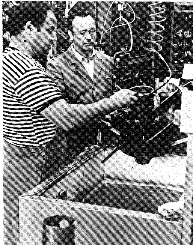
Precejšnjo pridobitev za tovarno je tudi korito za preizkus tesnosti zvarov. Precej lažje je upravljati z njim, od sodobnih naprav v svetu pa se razlikuje tudi po grelcu za vodo. Ta ima vse leto enako temperaturo, kar zmanjšuje tudi poklicne bolezni pri delavcih, ki delajo pri testiranju tesnosti ohišij grelcev. Tudi to napravo je konstruiral Anton Maček.
