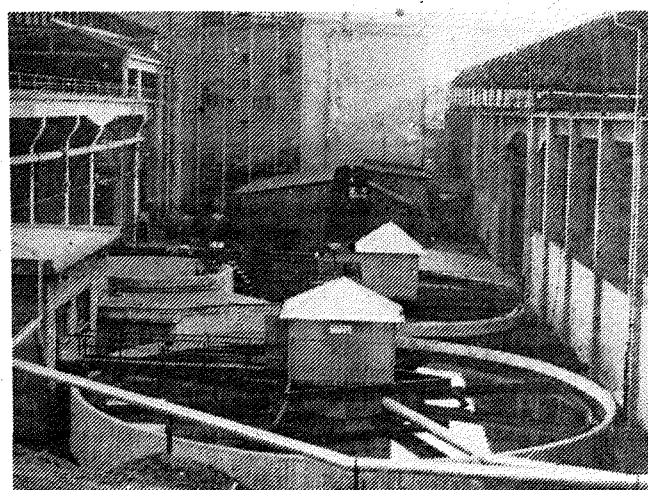
Nova čistilna naprava industrijskih voda v starih obratih Železarne Štore, 1982
