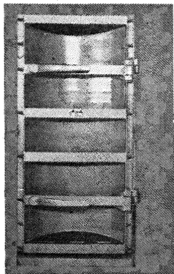
Vrata, odporna proti tlaku (VHP 0,9 MPa) in hermetična
