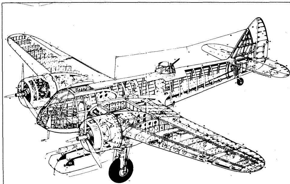
Risba »slečenega« Bristol Blenheima Mk I. Največja hitrost 426 km/h, največja potovalna hitrost 370 km/h, najboljša ekonomska hitrost 265 km/h (vse na višini 4575 m = 15.000 čevljev), doseg 1480 km pri 265 km/h, vzletna pot 713 m čez ovire 15 m. Teža 5013 kp, s tovorom 5947 kp, razpon 17,17 m, dolžina 12,12 m, višina 3,89 m. Desno za pilotskim sedežem je prostor za navigatorja (bombardierja), v sredini trupa pa za radijskega operaterja/strelca. (Po AIR ENTHUSIAST/SIXTEEN, risba Pilot Press – Aviagraphics; vizirnik je seveda tudi vseh 125 pojasnil za posamezne dele letala)
