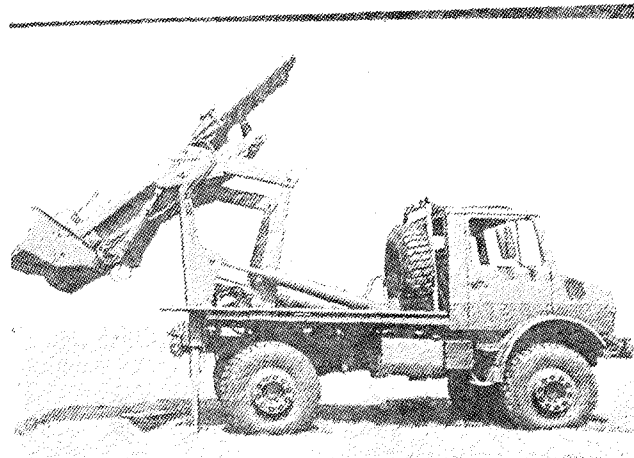
S pomočjo hidravlike voznik postavi okvir z minometnimi cevmi na tla.
