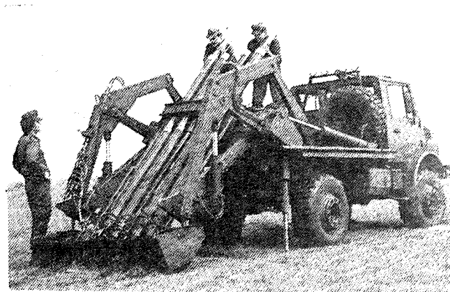
Potem ko je voznik in komandir vnesel vse potrebne podatke, strežaka napolnita cevi.
