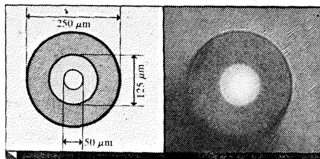
Takšen je prerez optičnega vlakna: sredica steklena, obdana še z drugim slojem (drugačnega) stekla, oblečenega v varovalni ovoj iz različnih zaščitnih mas (plastike, teflona...)
