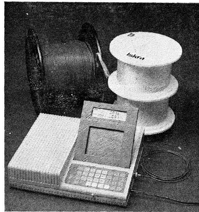
Tukaj je predstavljen le del proizvodnje Elektrooptike; poleg optičnih vlaken je naprava za digitalni optični reflektometer, ki je potreben za kontrolo poti svetlobe po kablu.
