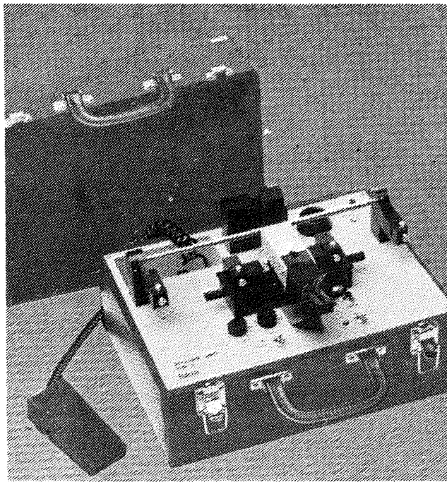
Spet ena izmed naprav, ki so jih v Elektrooptiki skonstruirali sami. Namenjena je pa izredno natančnemu »varjenju« – spajanju posameznih delov optičnih kablov (vlaken v kablji).
