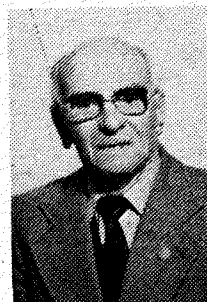
Franc Kurnik
