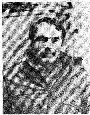
Polde Kožar
