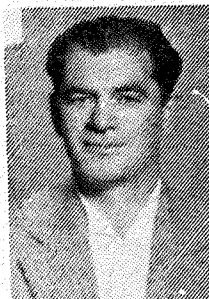
BoŹidar Cvek
