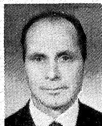
JoŹe Šobar
