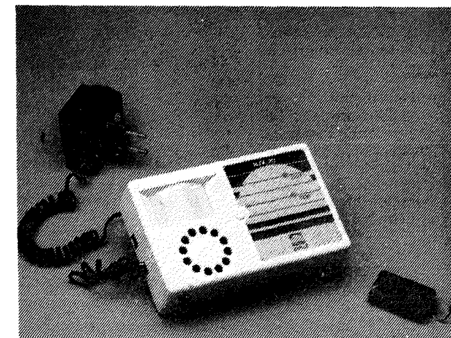
Elektronska naprava za javljanje vloma NJV-30, ki jo izdelujejo v montažnem podjetju Zarja v Kamniku.
