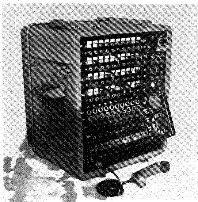
Prenosna telefonska centrala, ki jo skupaj izdelujeta Elektronska industrija iz Niša in Institut Mihajlo Pupin.
