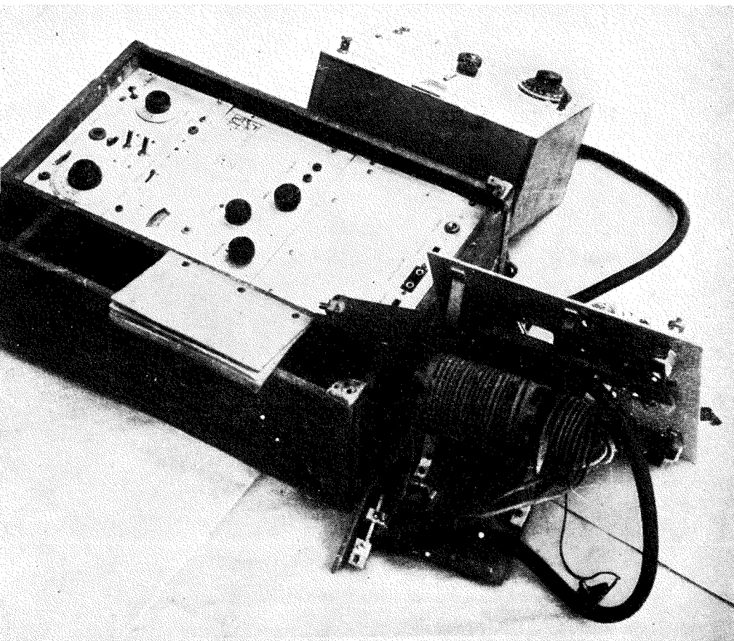
Ta fotografija predstavlja, po izjavah sodelavcev »Kričača«, približno kopijo aparature, ki so jo uporabljali pri oddajanju v Ljubljani
