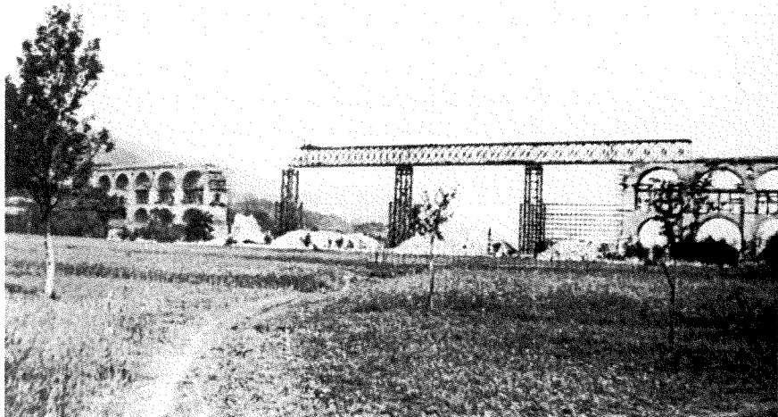
Obnova Borovniškega mostu po prvem rušenju 1941.
